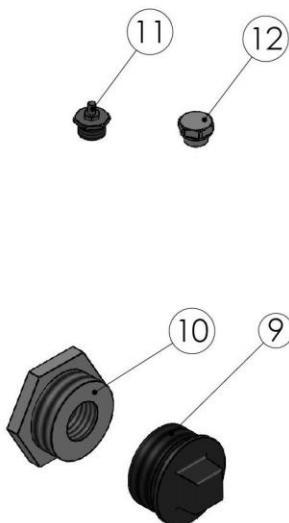
Rys. 5 Osprzęt zbiornika hydroforowego - HVP leżący
