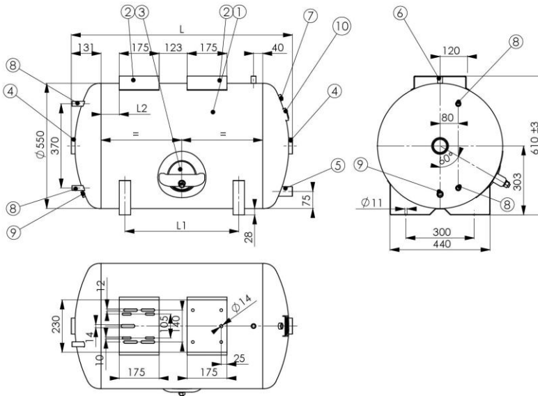
Rys.2 Zbiornik hydroforowy - HVP201L / HVP301L
